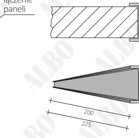
Ochroniacz krawędzi
