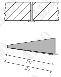
Łącznik czołowy
