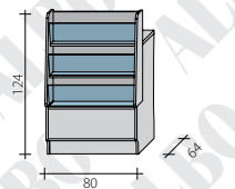
Lada pełna -80 gazeciarnz wysoki
