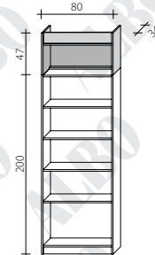
Nadstawka prosta do R-80
