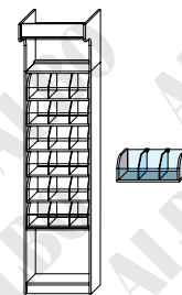
Półka cukiernicza do R-60
