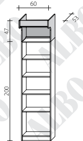
Nadstawka baldachimowa do R-60 z oświetleniem GZ1
