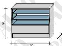
Łada przeszklona w 2/3 - 120
