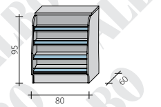
Lada pełna -80 z impulsem niskim
