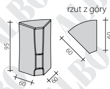
Lada narożna wewnętrzna 45 stopni
