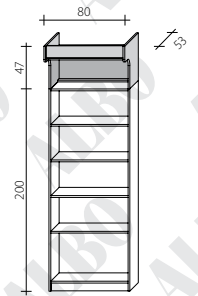
Nadstawka baldachimowa do R-80 z oświetleniem GZ1
