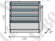
Lada pełna -120 z impulsem wysokim
